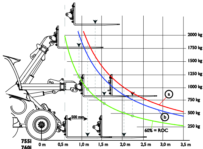
Diagrama de cargas de 755i / 760i
